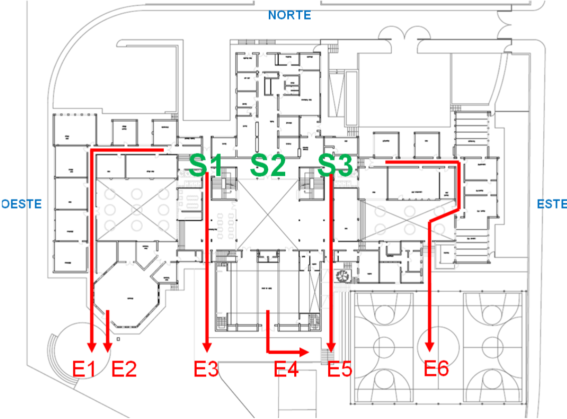
PLANTA BAJA
