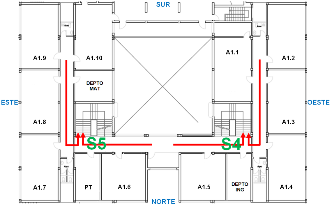
PLANTA PRIMERA
